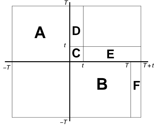
Figure 3. S_\Delta の積分領域
